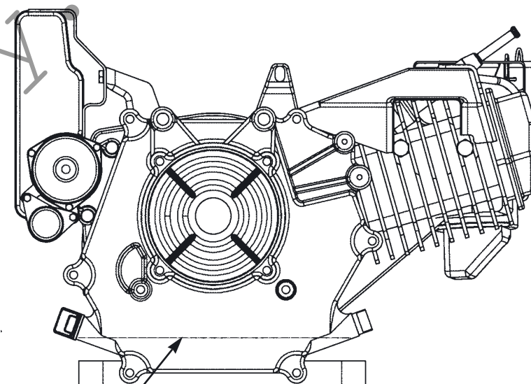
Уровень масла
